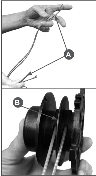
Рис. 17 Подготовка корда
